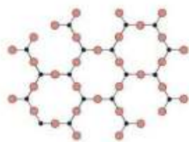
Estrutura Cristalina
